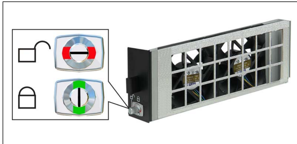
Figure 4: Lüftereinschub
